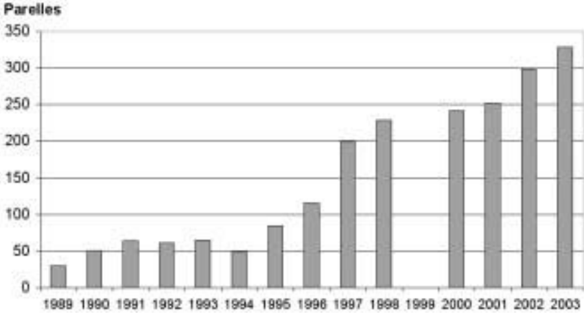
Gràfic 3.- Evolució numèrica dels totals de parelles d'ardeids que han criat a s'Albufera. L'any 1999 no ni ha dades fiables. Figure 3. Numerical evolution of the breeding pairs in s'Albufera de Mallorca. The results of the year 1999 are not reliable.
